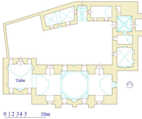
Melik Mansur Medresesi Planı (M. Baran Arşivi'nden)
